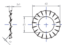
Forma A dentado exterior
