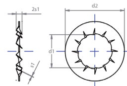
Forma J dentado interior
